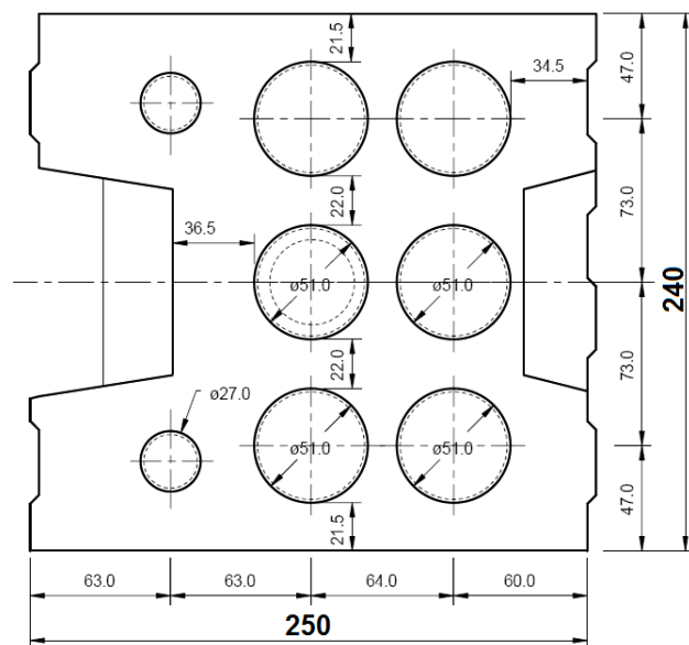
Fig. 3 KSL 12 8DF
