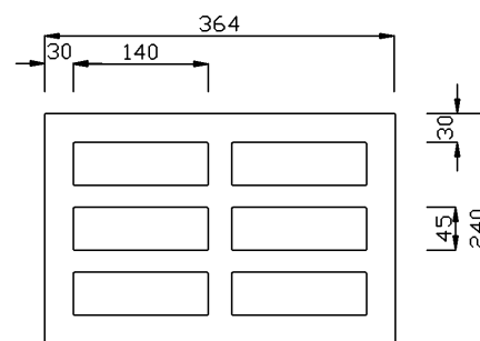
Fig. 6 HBN 1,4 16DF
