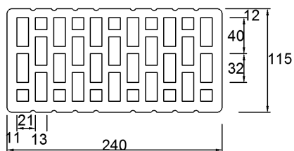
Fig. 1 HLZ 12 2DF
