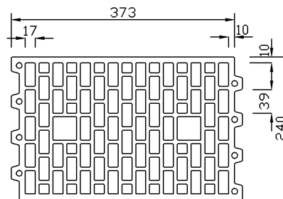
Fig. 2 HLZ 12 16DF
