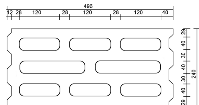
Fig. 5 HBL 2-0,8 16DF
