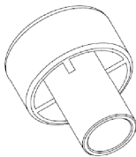
Verfüllstutzen VS Bohrerdurchmesser ( d_0 ): 18 mm bis 40 mm
