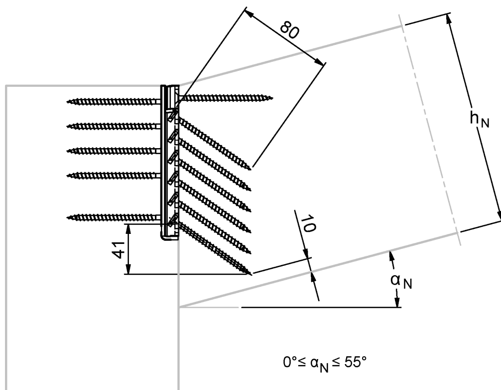
Ansicht
