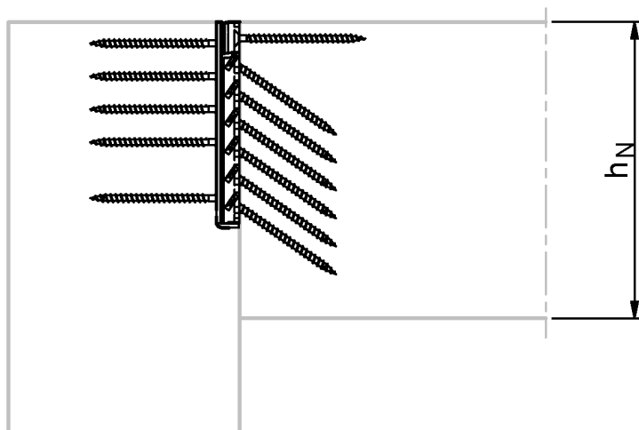
Ansicht
