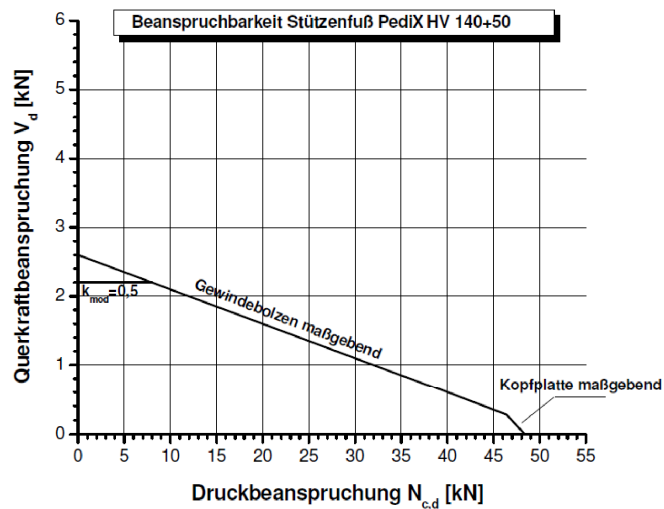
Abbildung B-2: Tragfähigkeiten des Stützenfußes PediX HV 140+50 bei Interaktion von Druck- und Querkraftbeanspruchungen für angenommene Teilsicherheitsbeiwerte \gamma_M = 1,3 , \gamma_{M0} = 1,0 , \gamma_{M1} = 1,1 und \gamma_{M2} = 1,25
