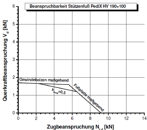
Abbildung B-3: Tragfähigkeiten des Stützenfußes PediX HV 190+100 bei Interaktion von Zug- und Querkraftbeanspruchungen für angenommene Teilsicherheitsbeiwerte \gamma_M=1,3 , \gamma_{M0}=1,0 , \gamma_{M1}=1,1 und \gamma_{M2}=1,25
