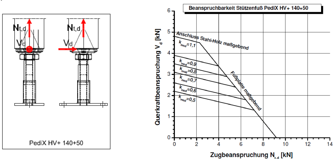
Abbildung B-5: Tragfähigkeiten des Stützenfußes PediX HV+ 140+50 bei Interaktion von Zug- und Querkraftbeanspruchungen für angenommene Teilsicherheitsbeiwerte \gamma_M = 1,3 , \gamma_{M0} = 1,0 , \gamma_{M1} = 1,1 und \gamma_{M2} = 1,25
