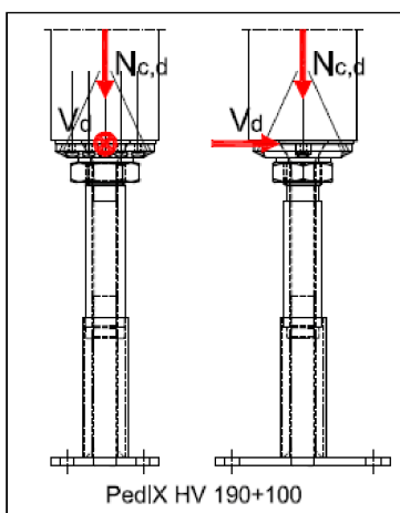
Abbildung B-4: Tragfähigkeiten des Stützenfußes PediX HV 190+100 bei Interaktion von Druck- und Querkraftbeanspruchungen für angenommene Teilsicherheitsbeiwerte \gamma_M=1,3 , \gamma_{M0}=1,0 , \gamma_{M1}=1,1 und \gamma_{M2}=1,25
