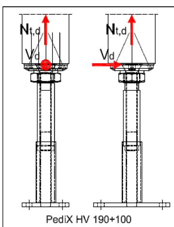
Abbildung B-3: Tragfähigkeiten des Stützenfußes PediX HV 190+100 bei Interaktion von Zug- und Querkraftbeanspruchungen für angenommene Teilsicherheitsbeiwerte \gamma_M=1,3 , \gamma_{M0}=1,0 , \gamma_{M1}=1,1 und \gamma_{M2}=1,25
