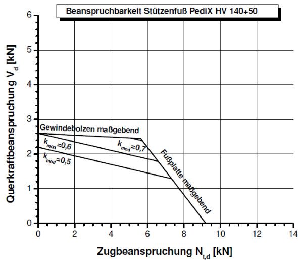
Abbildung B-1: Tragfähigkeiten des Stützenfußes PediX HV 140+50 bei Interaktion von Zug- und Querkraftbeanspruchungen für angenommene Teilsicherheitsbeiwerte \gamma_M = 1,3 , \gamma_{M0} = 1,0 , \gamma_{M1} = 1,1 und \gamma_{M2} = 1,25
