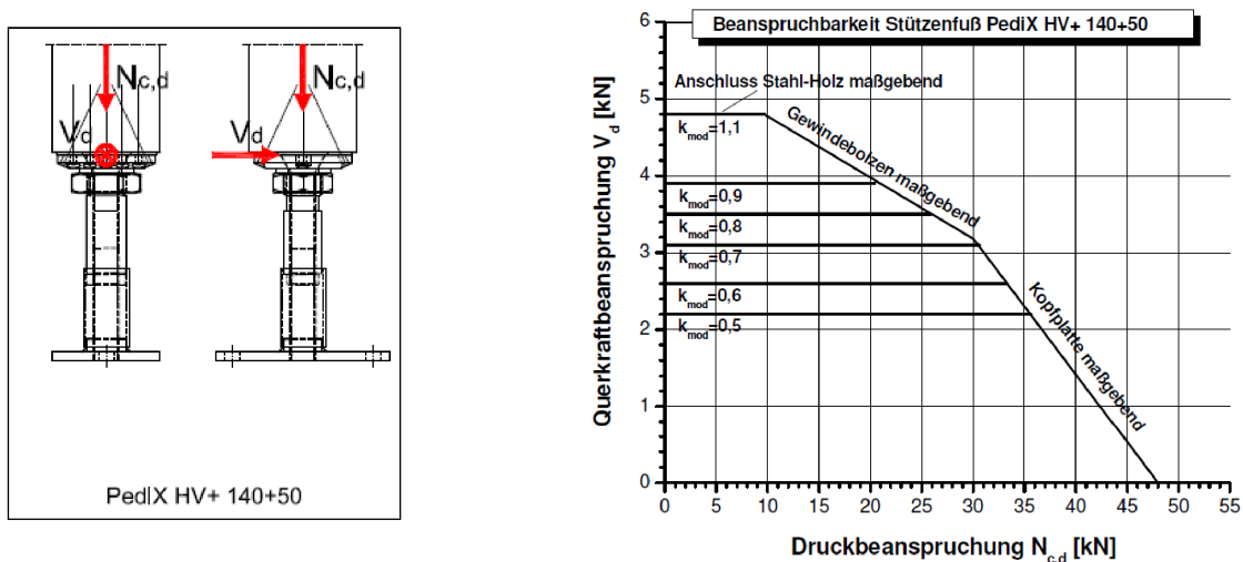
Abbildung B-6: Tragfähigkeiten des Stützenfußes PediX HV+ 140+50 bei Interaktion von Druck- und Querkraftbeanspruchungen für angenommene Teilsicherheitsbeiwerte \gamma_M = 1,3 , \gamma_{M0} = 1,0 , \gamma_{M1} = 1,1 und \gamma_{M2} = 1,25
