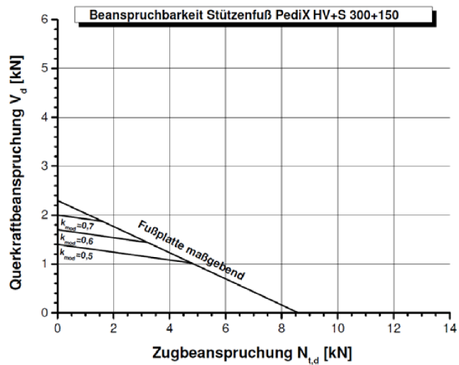
Abbildung B-9: Tragfähigkeiten des Stützenfußes PediX HV+S 300+150 bei Interaktion von Zug- und Querkraftbeanspruchungen für angenommene Teilsicherheitsbeiwerte \gamma_M=1,3 , \gamma_{M0}=1,0 , \gamma_{M1}=1,1 und \gamma_{M2}=1,25
