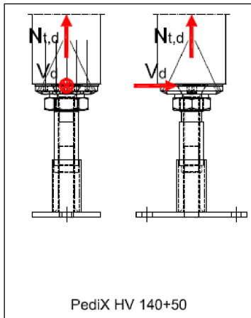
Abbildung B-1: Tragfähigkeiten des Stützenfußes PediX HV 140+50 bei Interaktion von Zug- und Querkraftbeanspruchungen für angenommene Teilsicherheitsbeiwerte \gamma_M = 1,3 , \gamma_{M0} = 1,0 , \gamma_{M1} = 1,1 und \gamma_{M2} = 1,25
