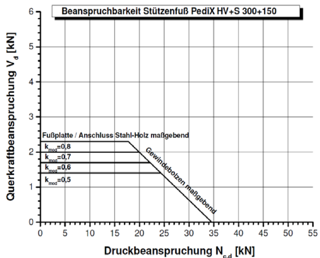
Abbildung B-10: Tragfähigkeiten des Stützenfußes PediX HV+S 300+150 bei Interaktion von Druck- und Querkraftbeanspruchungen für angenommene Teilsicherheitsbeiwerte \gamma_M=1,3 , \gamma_{M0}=1,0 , \gamma_{M1}=1,1 und \gamma_{M2}=1,25
