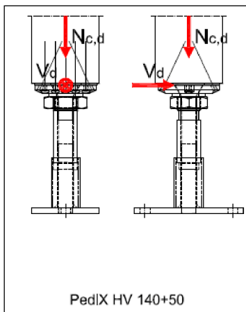
Abbildung B-2: Tragfähigkeiten des Stützenfußes PediX HV 140+50 bei Interaktion von Druck- und Querkraftbeanspruchungen für angenommene Teilsicherheitsbeiwerte \gamma_M = 1,3 , \gamma_{M0} = 1,0 , \gamma_{M1} = 1,1 und \gamma_{M2} = 1,25
