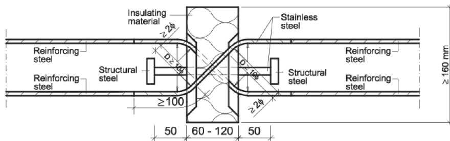
Fig. 20 Schöck Isokorb® type Q+Q with SCE
