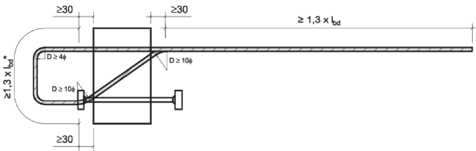
Fig. 44 Schöck Isokorb® type O
