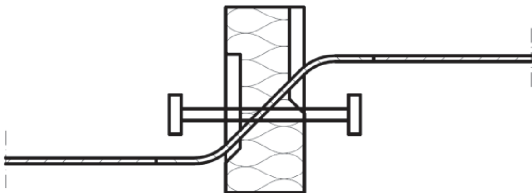
Fig. 4 Schöck Isokorb® type Q
