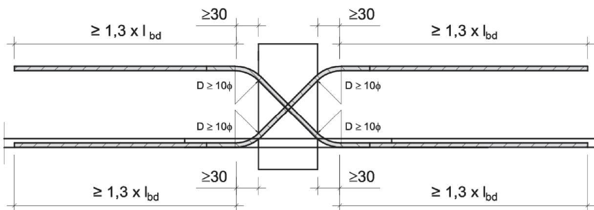
Fig. 40 Schöck Isokorb® type D
