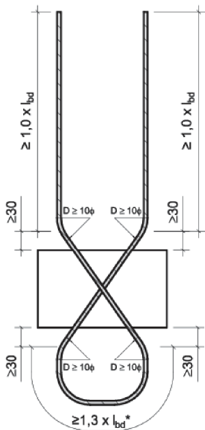
Fig. 42 Schöck Isokorb® type A
