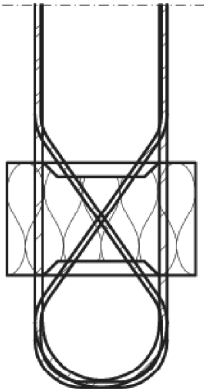
Fig. 7 Schöck Isokorb® type A
