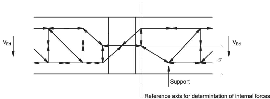
Fig. 36 Schöck Isokorb® type Q
