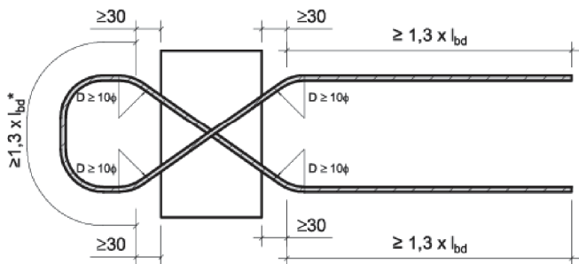
Fig. 42 Schöck Isokorb® type A
