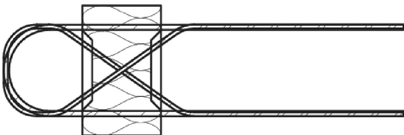
Fig. 7 Schöck Isokorb® type A
