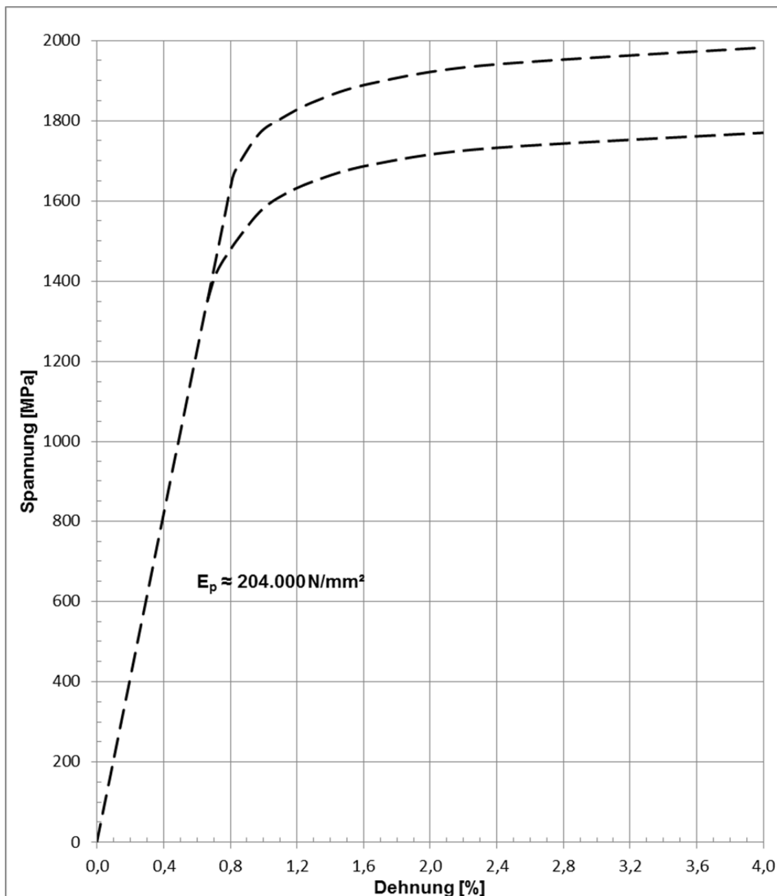
Bild 2: Prinzipieller Spannungs-Dehnungs-Verlauf
