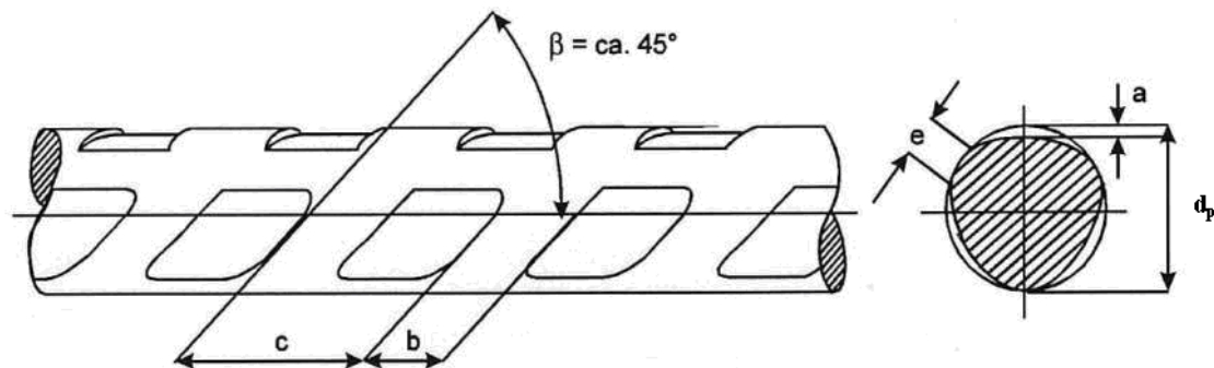
Bild 1: Ansicht des profilierten Spannstahldrahts
