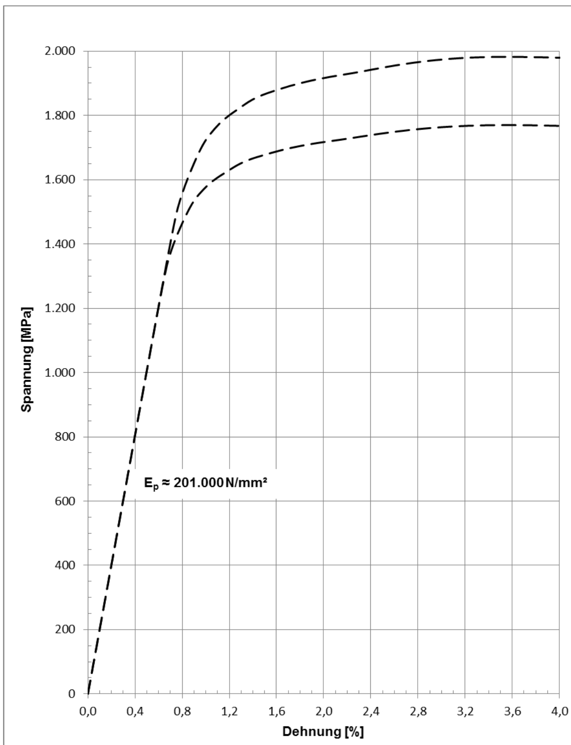
Bild 2: Prinzipieller Spannungs – Dehnungsverlauf
