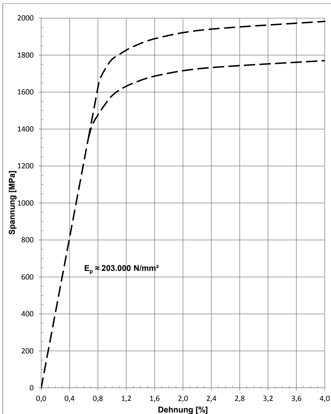
Bild 2: Prinzipieller Spannungs-Dehnungs-Verlauf
