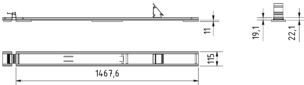
Detail: Bodenschiene
