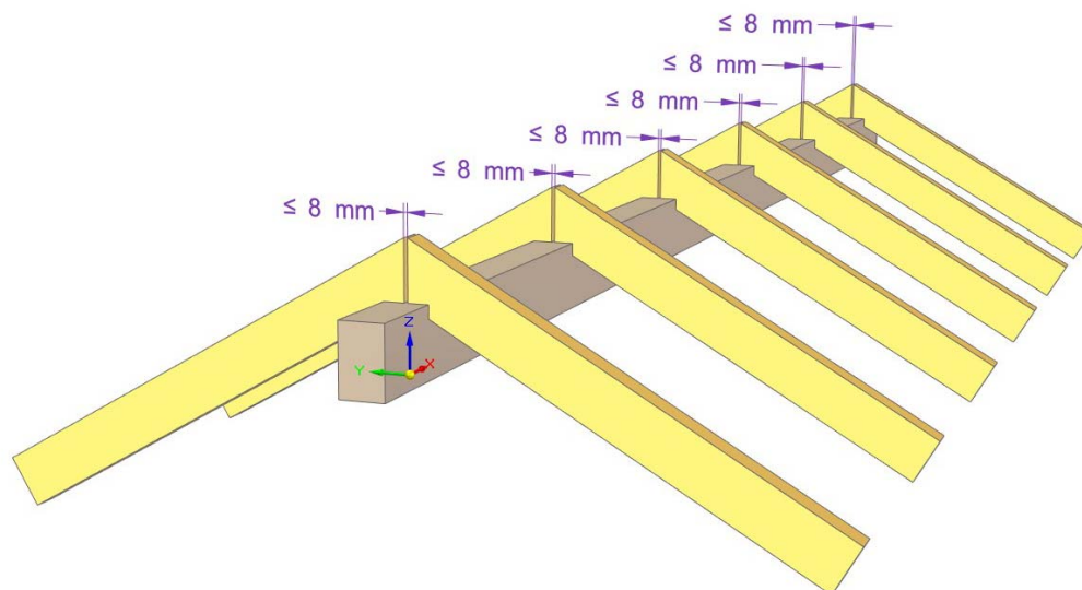
Abbildung 1 - maximales Spaltmaß am Sparrenstoß
