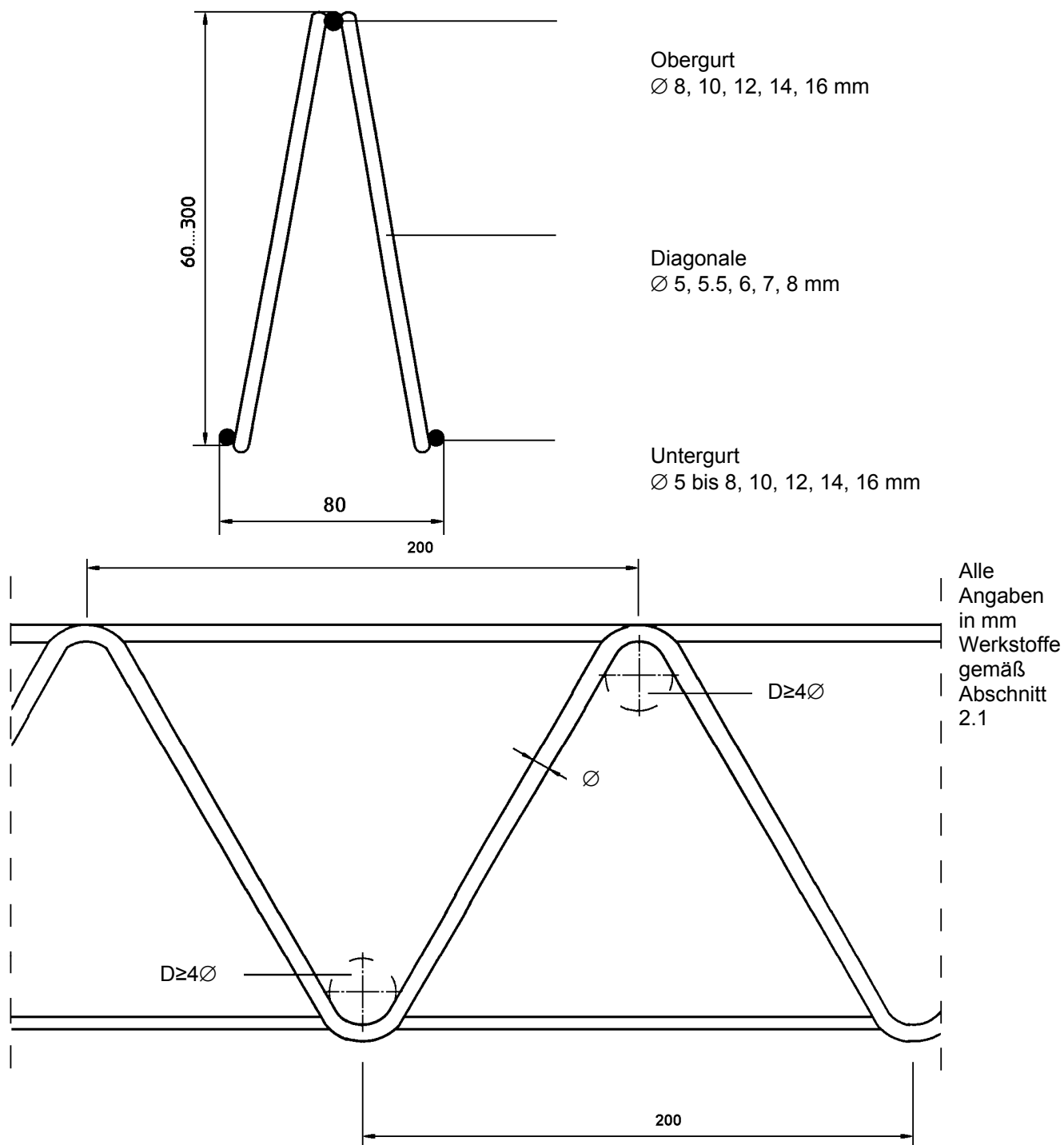
Bild 1: Darstellung des Gitterträgers
