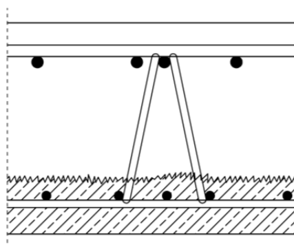
Bild 9: Gitterträger als Verbund- und Querkraftbewehrung (hohe Beanspruchung)
