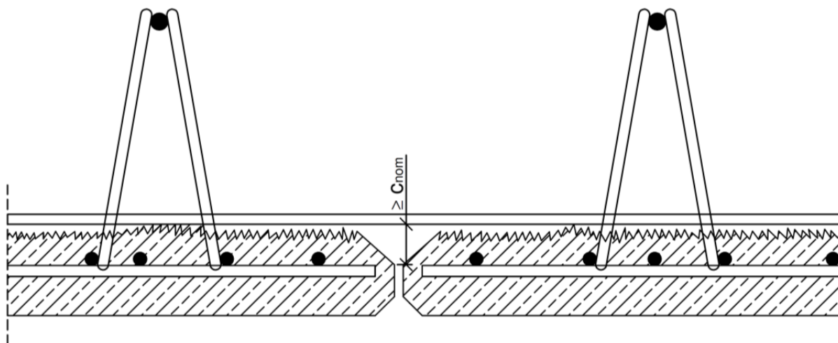
Bild 5: Abfasung an Elementrändern
