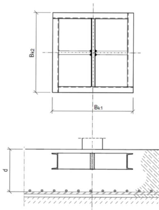
Bild 6.1: unter Betonstütze
