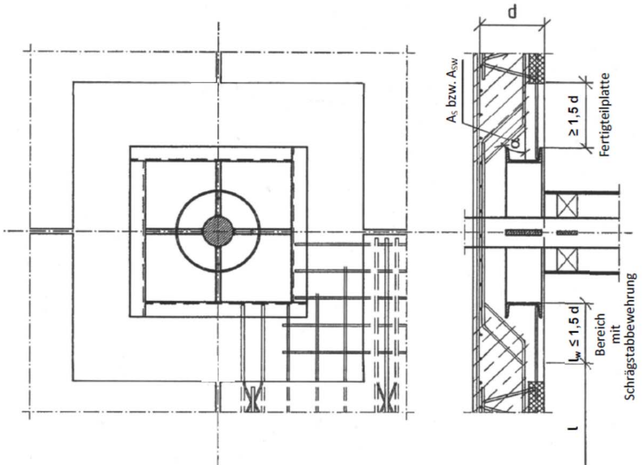
Bild 7: Beispiel für die Kombination mit einer Fertigteilplatte mit statisch mitwirkender Ortbetonschicht
