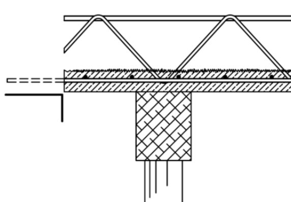
Bild 6: Auflagerung mit Montageunterstützung am Rand
