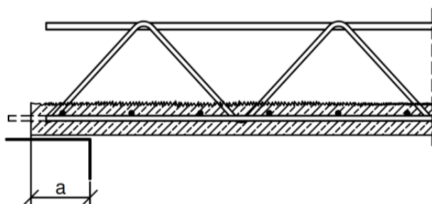
Bild 5: Auflagerung ohne Montageunterstützung am Rand
