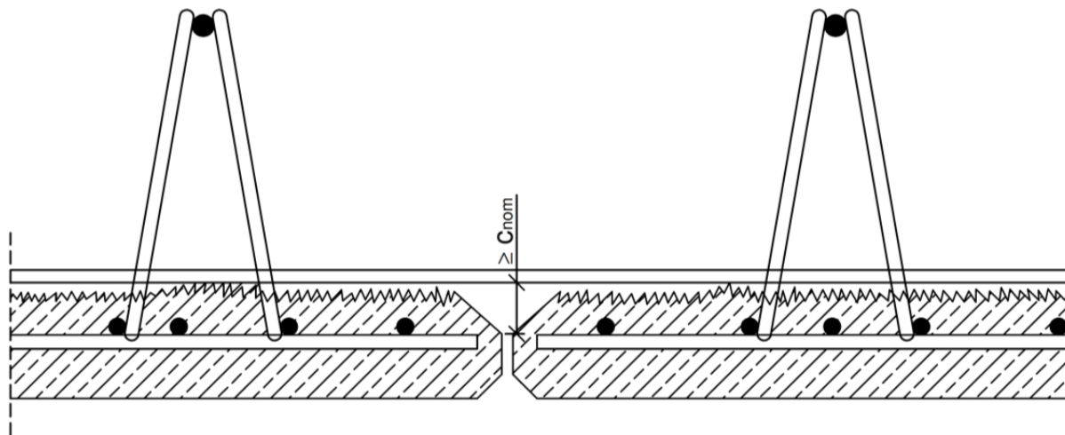
Bild 7: Abfasung an Elementrändern
