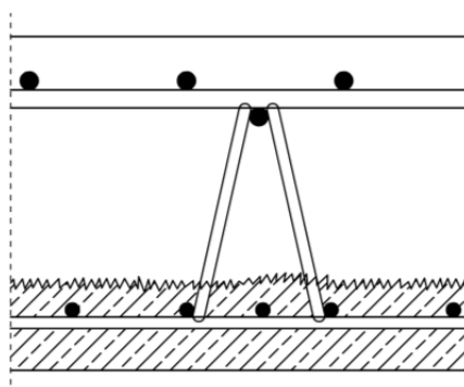
Bild 10: Gitterträger als Verbund- und Querkraftbewehrung (mäßige Beanspruchung)
