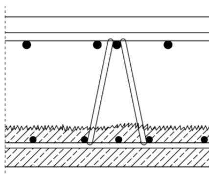
Bild 11: Gitterträger als Verbund- und Querkraftbewehrung (hohe Beanspruchung)
