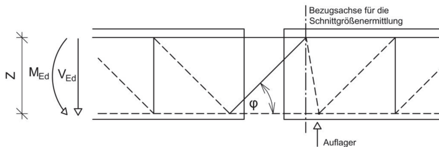
Typ A-MQ/B-MQ indirekte Stützung
