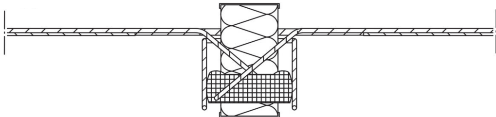
TYP ISOPRO A-MQQ
