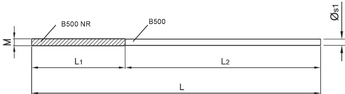
Bild 6: B500NR (L1 als Teil- oder Vollgewinde) mit B500
