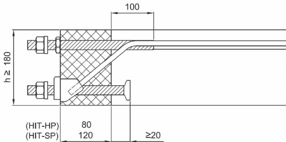
Bild 1: Halfen-Iso-Element HIT-HP/SP SDV mit Zug-/Druckstäben
