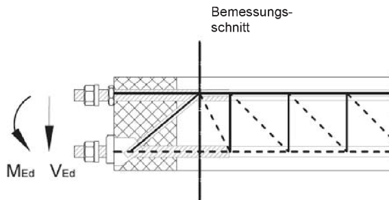
Bild 9: Fachwerkmodell HIT-HP/SP SDV mit Stahlfachwerk (SMV analog)
