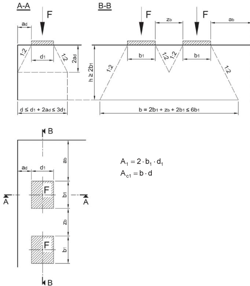
Bild 11: Bestimmung der rechnerischen Verteilerfläche A_{c1} nach Leonhardt (Vorlesung über Massivbau – Teil 2: Sonderfälle der Bemessung im Stahlbetonbau)
