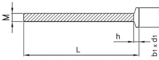
Bild 7: Druckstab aus nichtrostendem Rundstahl S690 bzw. A4-80 oder B500 NR jeweils mit Teil- oder Vollgewinde mit Kopfbolzen bzw. mit angeschweißter Ankerplatte S235
