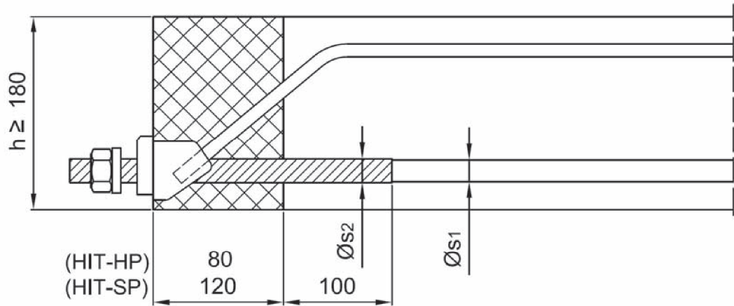
Bild 3: Halfen-Iso-Element HIT-HP/SP SZV mit Druckstab
