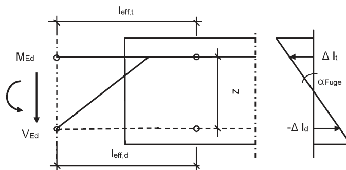
Bild 13: Modell für die Ermittlung der Biegeverformungen in der Fuge
