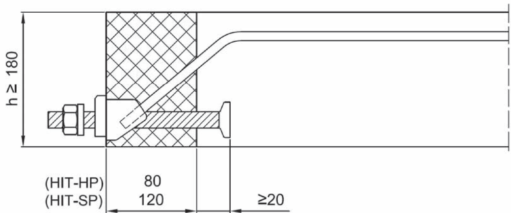
Bild 4: Halfen-Iso-Element HIT-HP/SP SZV, Variante mit Kopfbolzen als Druckstab
