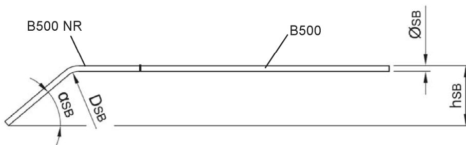
b) Ausführung nichtrostender Betonstahl B500 NR mit B500
