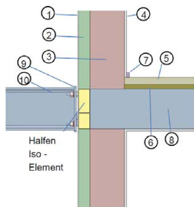
Bild 14: Wandaufbau mit Wärmedämmung
