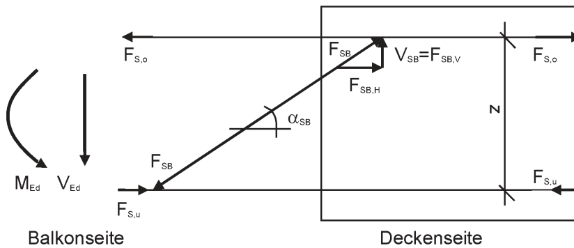
Bild 10: Fachwerkmodell HIT-HP/SP SDV/SMV
