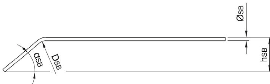
a) Ausführung nichtrostender Betonstahl B500 NR
