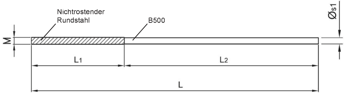
Bild 5: Standardausführung aus nichtrostendem Rundstahl S690 bzw. A4-80 (L1 als Teil- oder Vollgewinde) mit B500
