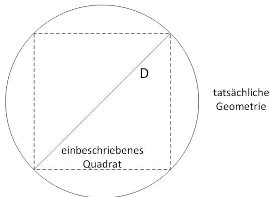
Abbildung 1: Ansetzbare Fläche bei runden Lagern zur Ermittlung des Formfaktors S mod
