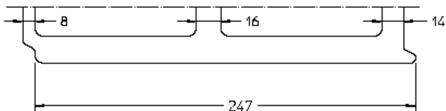
alternativer Außenlängssteg
