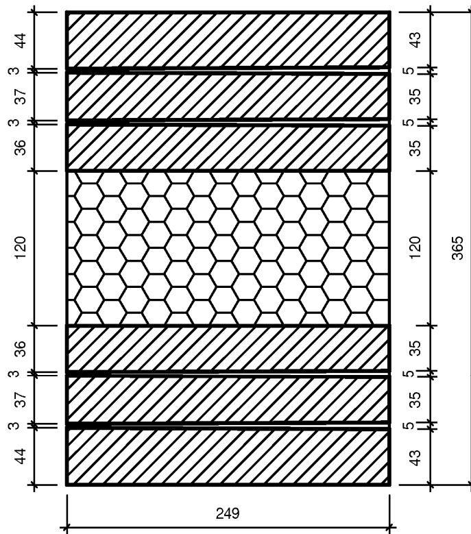
Schnitt B-B
