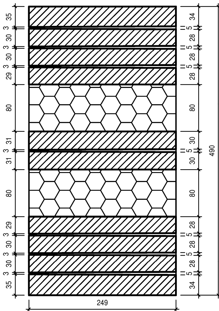
Schnitt B-B
