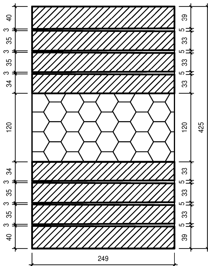
Schnitt B-B
