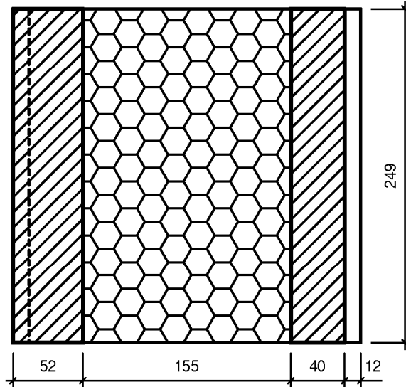
Schnitt B-B
