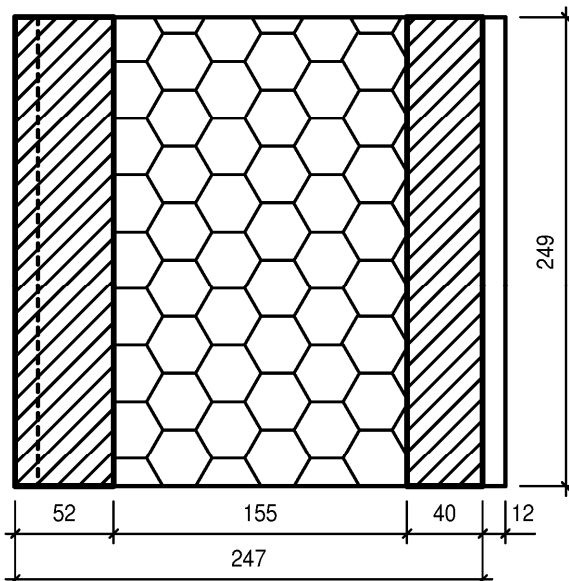
Schnitt B-B
