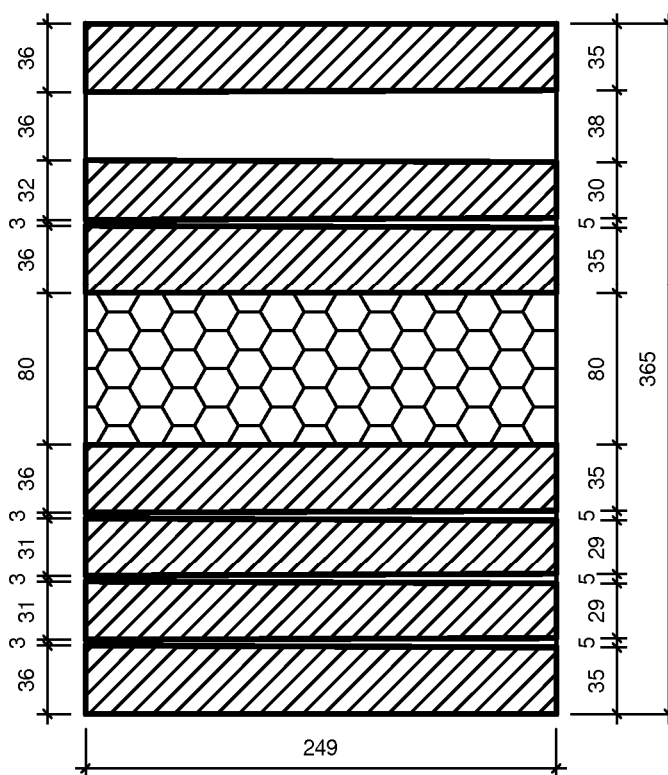
Schnitt B-B
