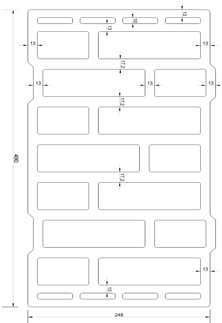
Die angegebenen Stegdicken sind Mindestwerte in mm
