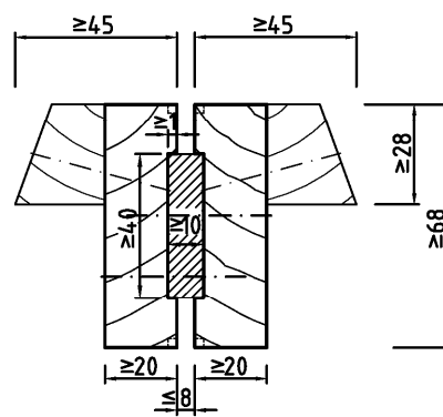
Schattennut-Verbindung
