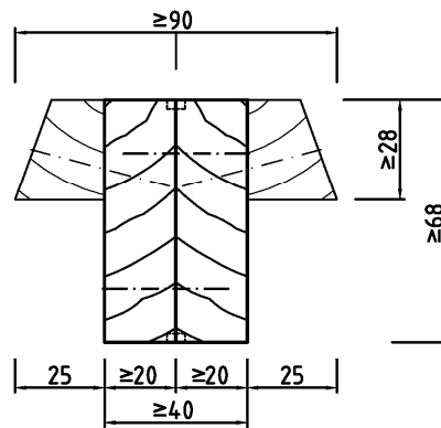
Stumpf-Verbindung
