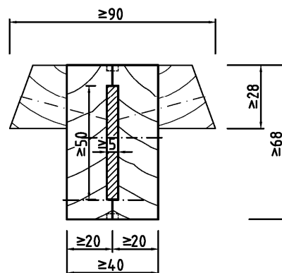
Flachfeder-Verbindung
