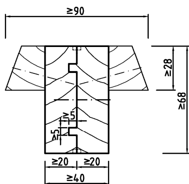
Zapfen-Verbindung
