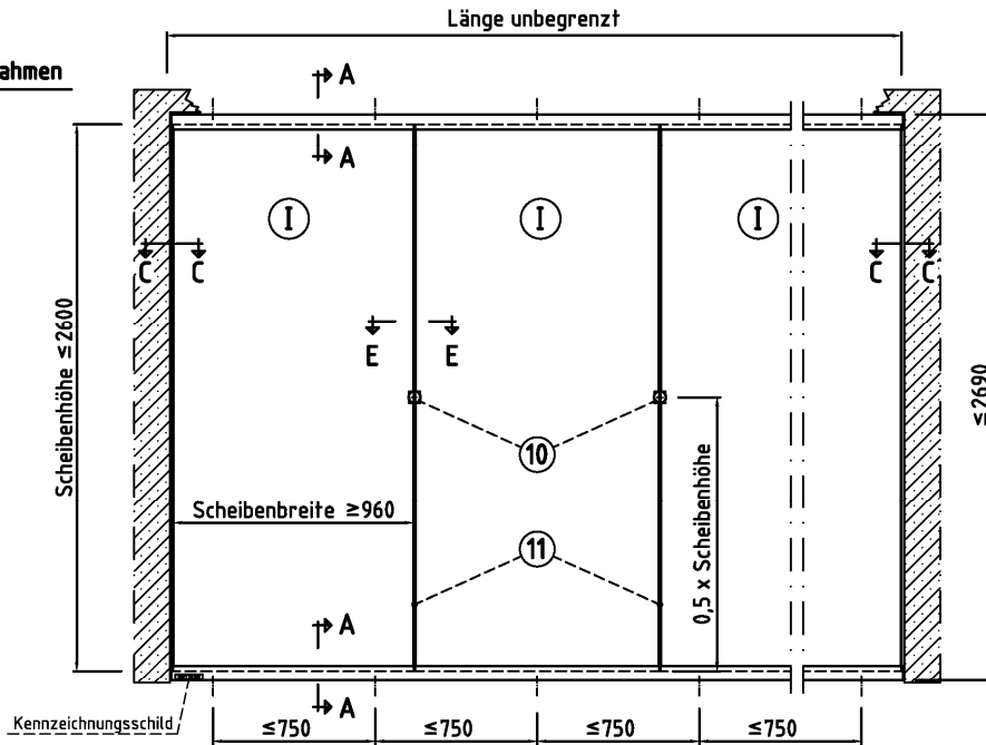
Ⓛ Maximal zulässige Abmessungen der "PYRAN ® S"-Glasscheiben:
