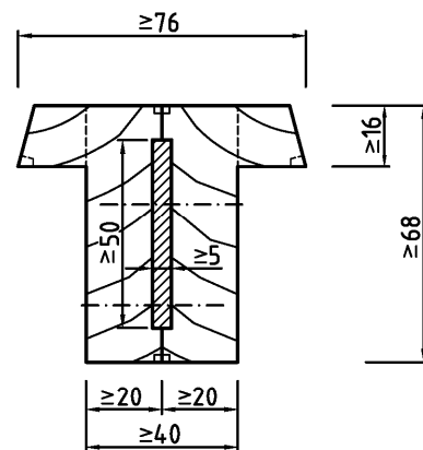
Flachfeder-Verbindung
