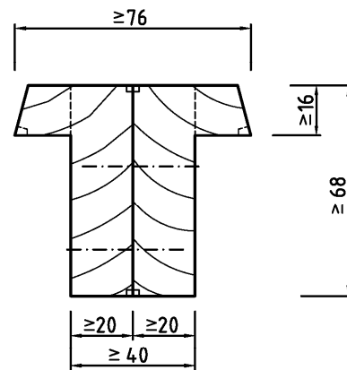
Stumpf-Verbindung
