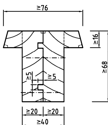
Zapfen-Verbindung
