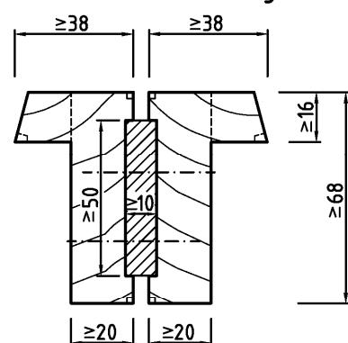
Schattennut-Verbindung
