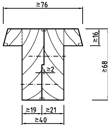
Falz-Verbindung
