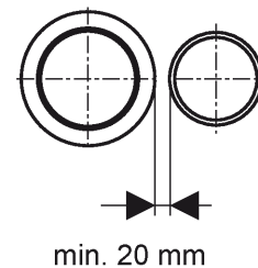
Lüftungsleitungen und Falleitungen kombiniert
