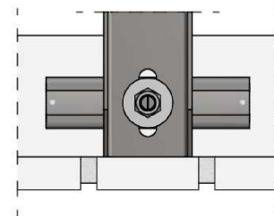
Anschlusskonstruktion mit einer Verschraubung
