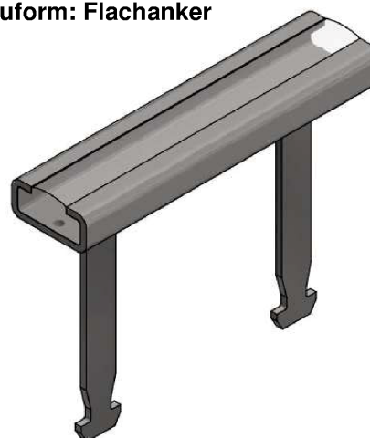
Bauform: Flachanker
