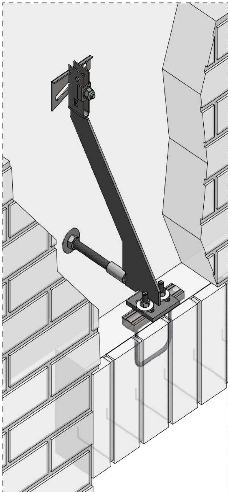
Bauform: Rundanker
