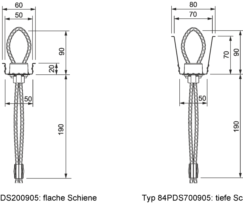
Bild 4: Verwahrkasten mit Seilschlaufe – Querschnitt
