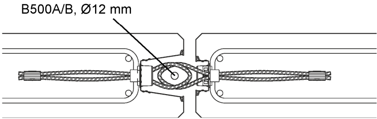
Bild 14: Anschluss Wand – Wand, Längsanschluss
