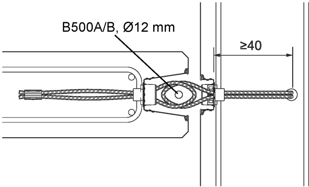
Bild 15: Anschluss Wand – Wand, Queranschluss
