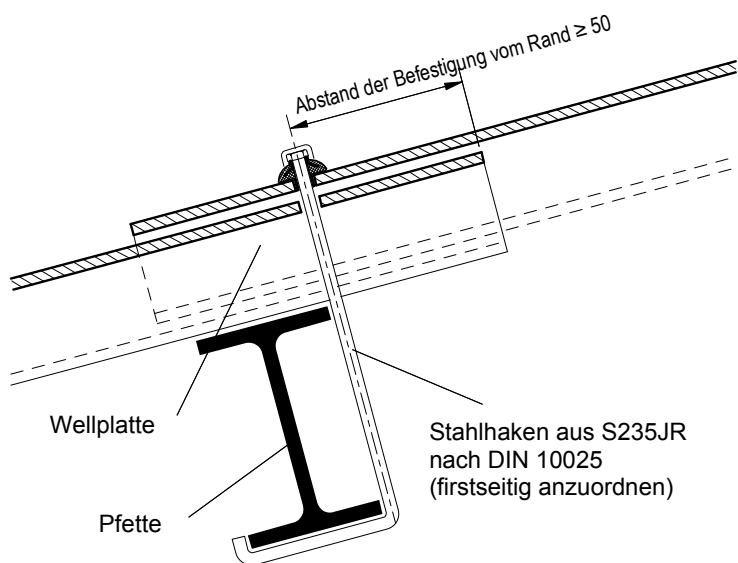
Anordnung der Befestigung mit Stahlhaken auf Stahl-Unterkonstruktionen
