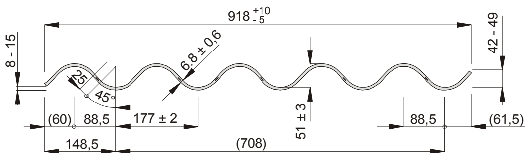
Bild 1.1: Wellplatte "Cembrit W177-5,5 RC" (Profil 5) mit PP-Bändern; Querschnittsabmessung und Lage der PP-Bänder
