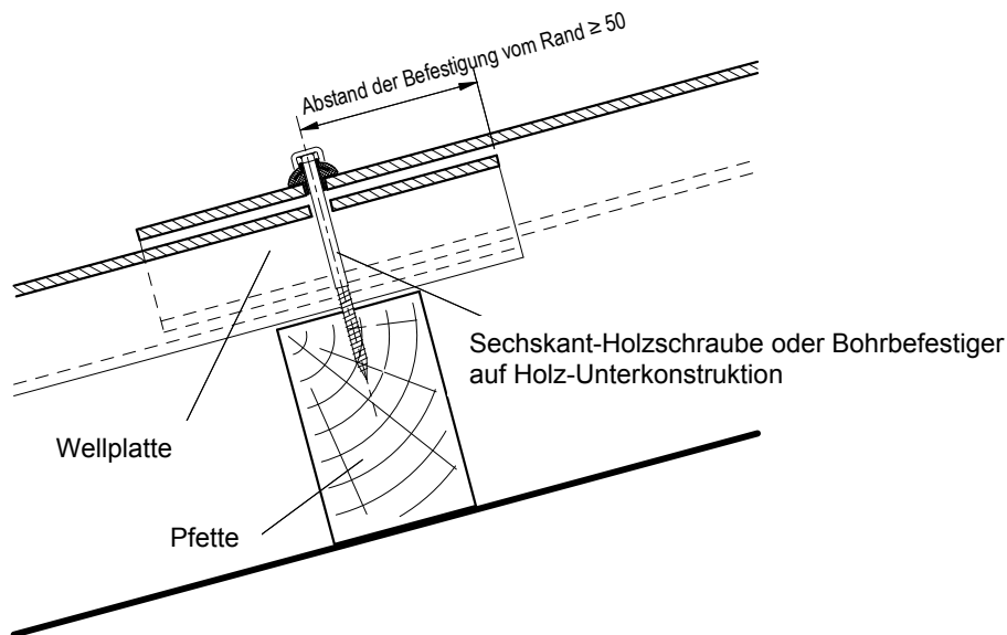
Anordnung der Befestigung auf Holz-Unterkonstruktionen
