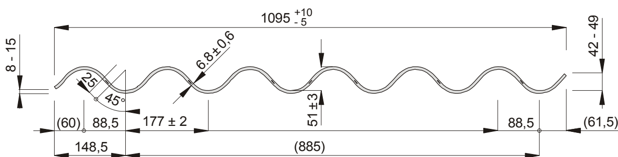
Bild 1.2: Wellplatte "Cembrit W177-6,5 RC" (Profil 6) mit PP-Bändern; Querschnittsabmessung und Lage der PP-Bänder
