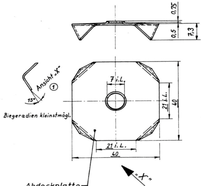
Abdeckplatte Bl. 1,5 DIN 1541-St Oberfläche galv. verzinkt!
