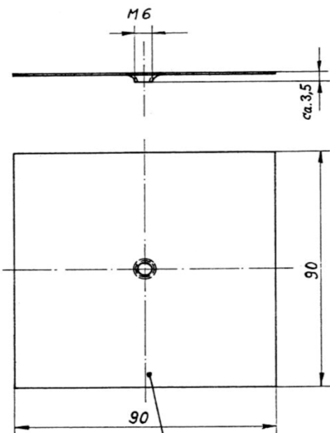
Gewindeplatte groß Bl. 1,5 DIN 1541-St Oberfläche galv. verzinkt!
