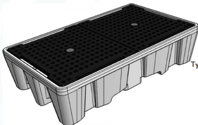
Typ C3 (Doppelstation mit Mittelstütze und Lochplatte, 1000 l)
