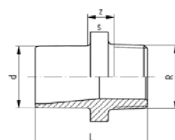
1.8: Übergangsnippel R / NPT (1.5 oben)
