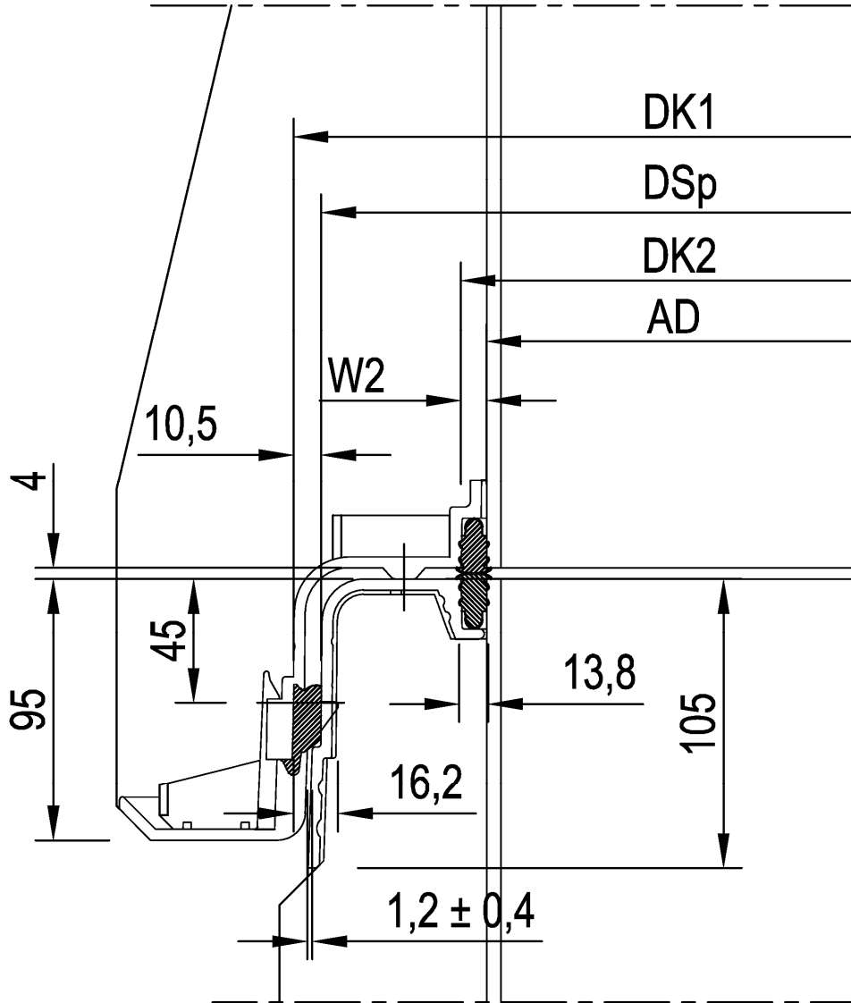
PP-B ausgekl. Rohrfügung, abwinkelbar, scherlastsicher u. schlagzäh
