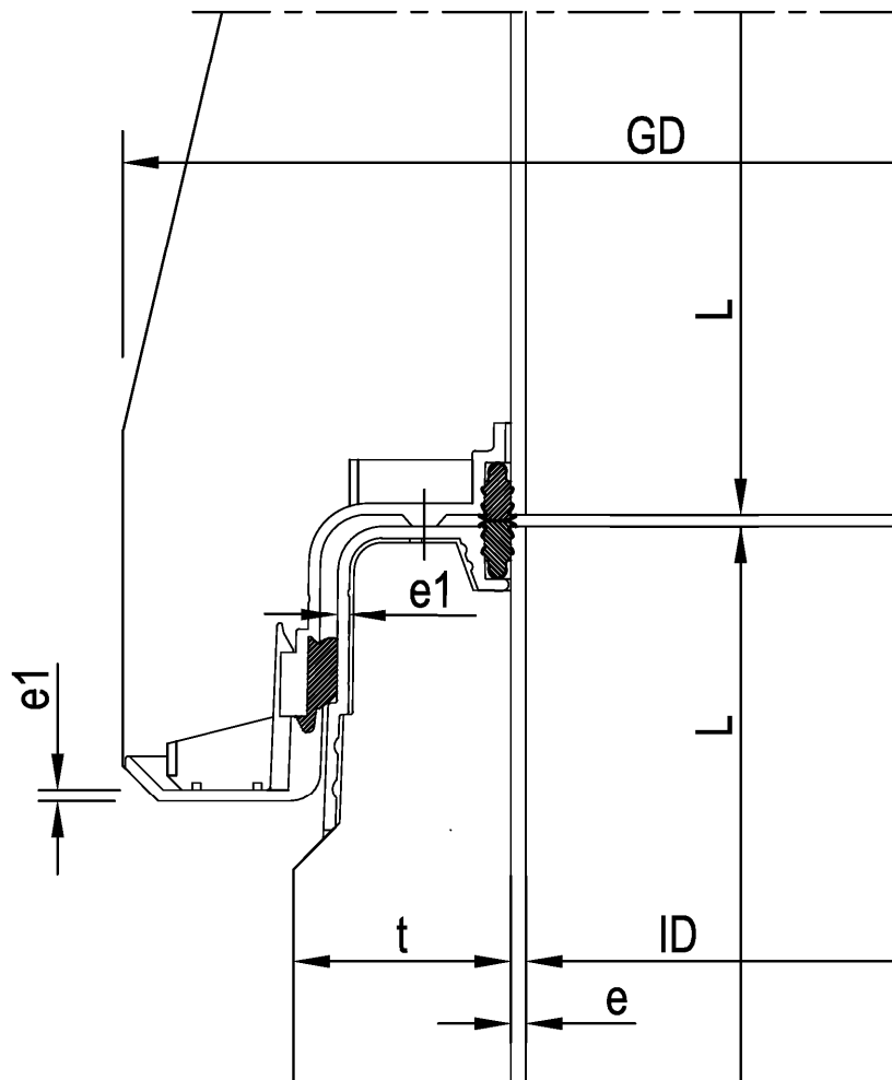
Beton- bzw. Stahlbeton/Polymer-Zweischichtrohr
