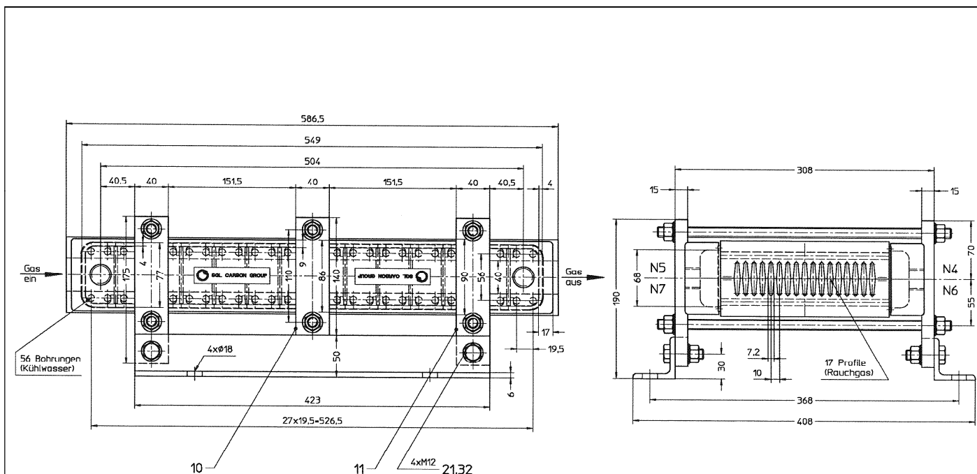
Draufsicht
