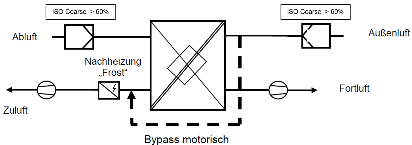
Anlagenschema – ValloPlus 270 SE und MV
