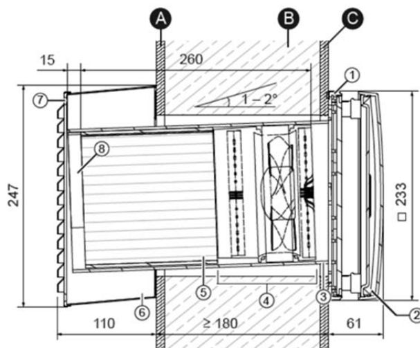
Schnittzeichnung Lüftungsgerät iV-Smart*, Variante Ohio
