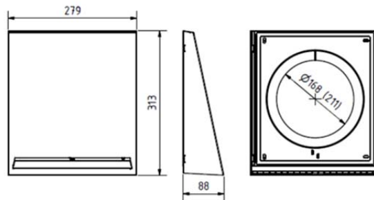
Grundplatte Wetterschutzhaube (ASA)
