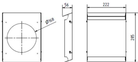
Grundplatte Wetterschutzhaube (Edelstahl)
