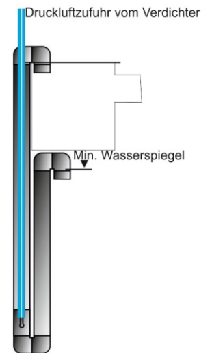
Klarwasserheber
