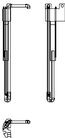
Belüfter einfach
