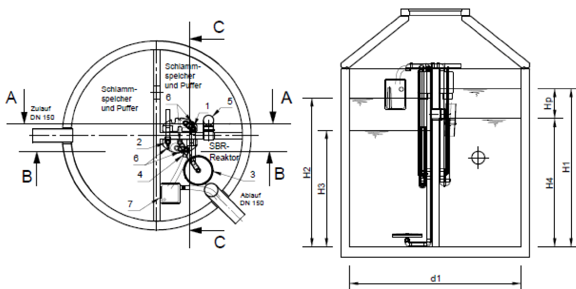
Schnitt C-C
