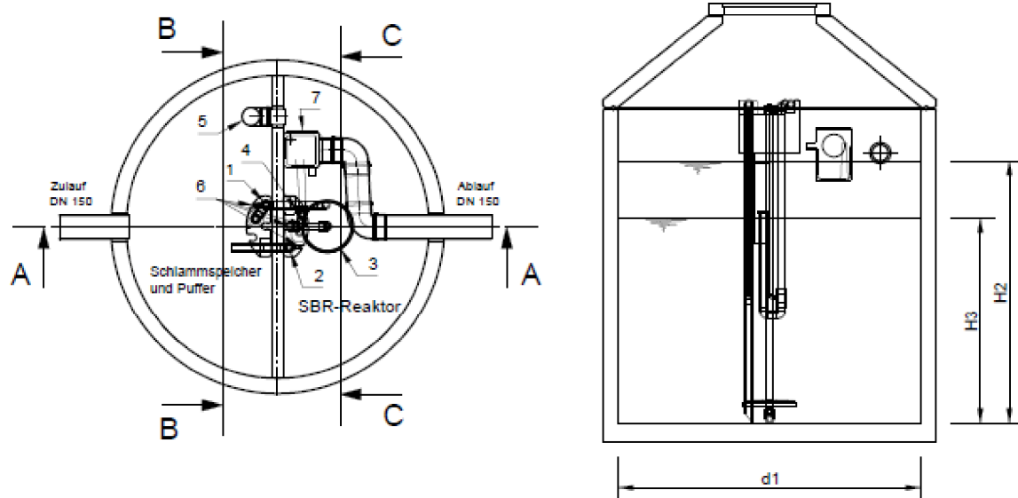
Schnitt C-C
