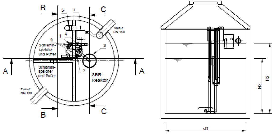
Schnitt C-C
