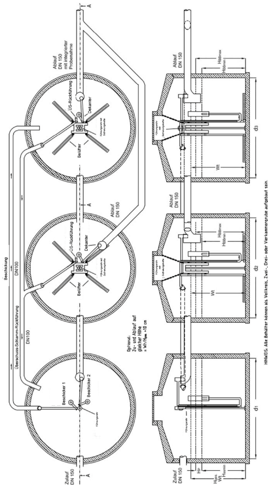
Nachrüstsatz Typ B&P SBR-Vario-Modul für den Einbau in bestehende Abwasserbehandlungsanlagen zur Herstellung von Kleinkläranlagen von 4 bis 50 EW; Ablaufklasse D
