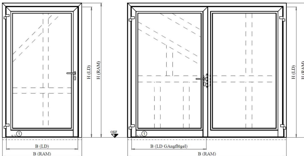
① Kennzeichnungsschild
