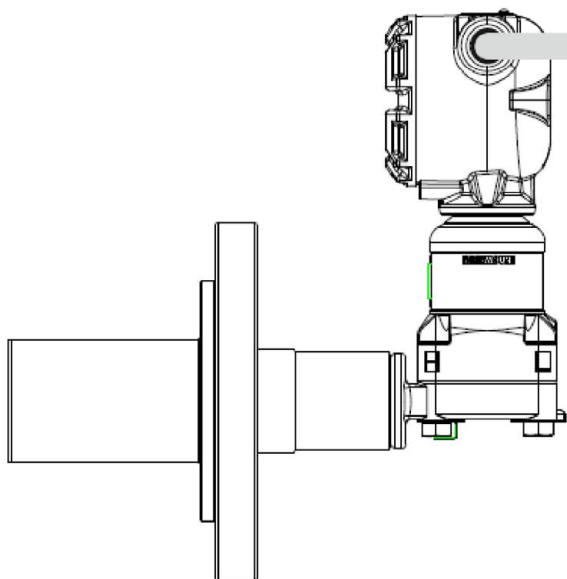
Sekundärgerät: 3051SAL Inline mit Druckmittler Typ EFW Direktanbau
