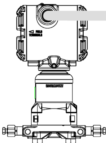
Sekundärgerät: 3051SAM Coplanar mit Anpassungsflansch
