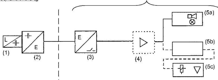
Schema der Überfüllsicherung
