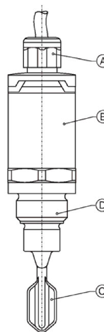
Liquiphant mit Kabelschwanz-Version
