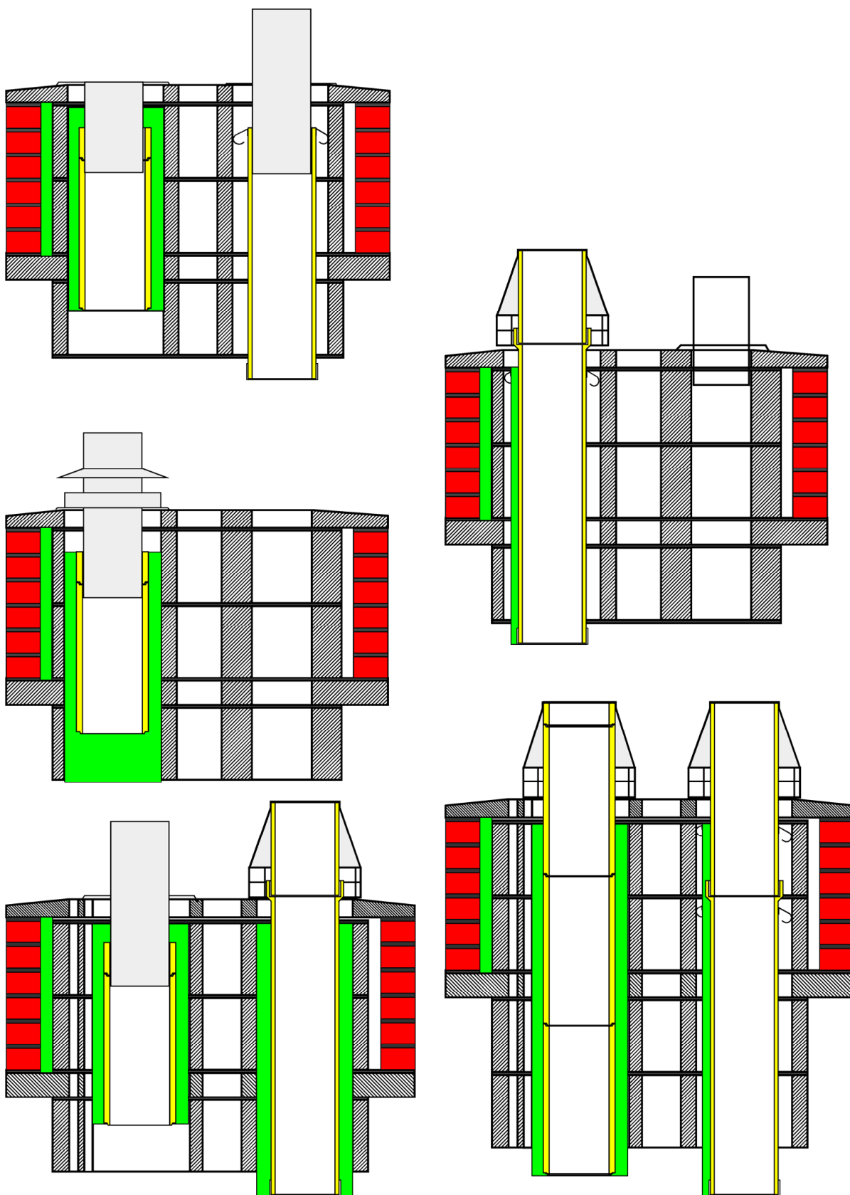
Bauarten für Bausätze aus Einzelteilen zur bauseitigen Montage von Abgasanlagen
