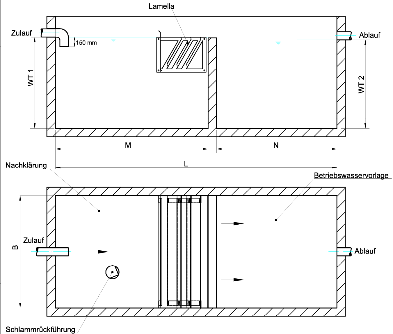
Nachklärung/Betriebswasservorlage in eckiger Ausführung
