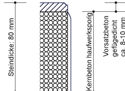
Schnitt (Randausschnitt)
