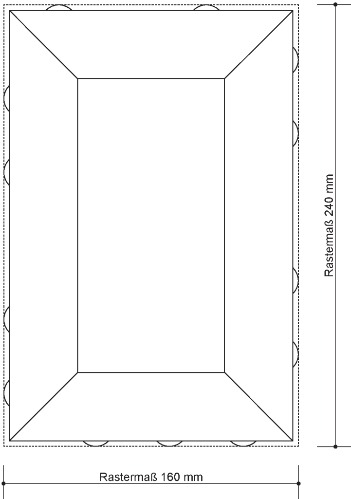
Draufsicht Betonpflasterstein 240/160/80 mm
