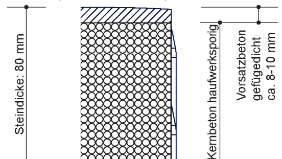
Schnitt (Randausschnitt)
