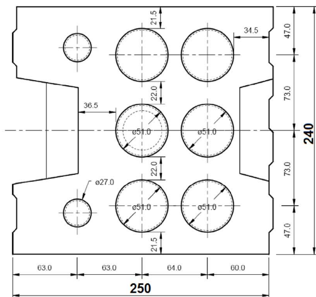
Bild 3 KSL 12 8DF
