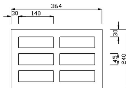
Bild 6 HBN 1,4 12DF
