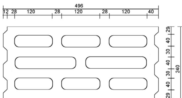
Bild 5 HBL 2-0,8 16DF
