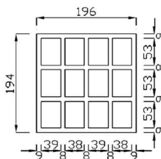
Bild 7 Brique Creuse C
