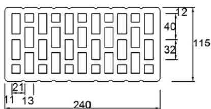
Bild 1 HLZ 12 2DF
