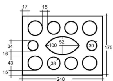
Bild 4 KSL 12-1.4 – 3DF
