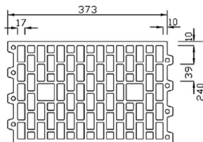
Bild 2 HLZ 12 12DF
