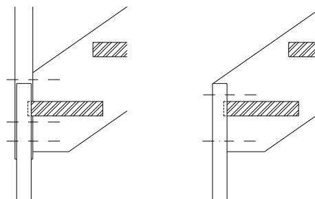
String-corner-joint
