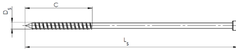
Spezialnagel S
