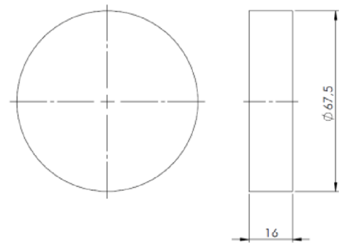
Dämmstofffrondelle
