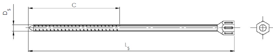
Spezialnagel PA
