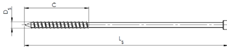
Spezialnagel S
