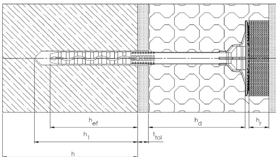
VERSENKTE MONTAGE
