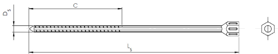
Spezialnagel PA
