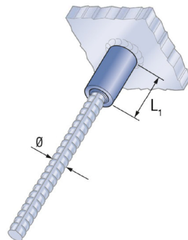
Fig. C9: PH-AH + PH-A
