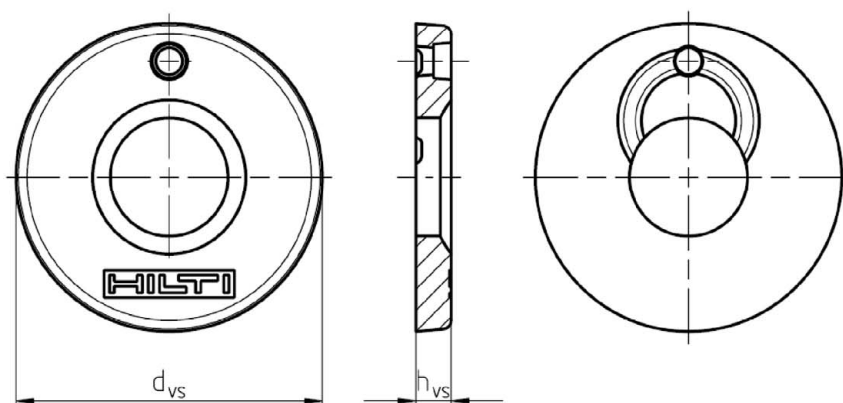
Hilti Verschlusscheibe
