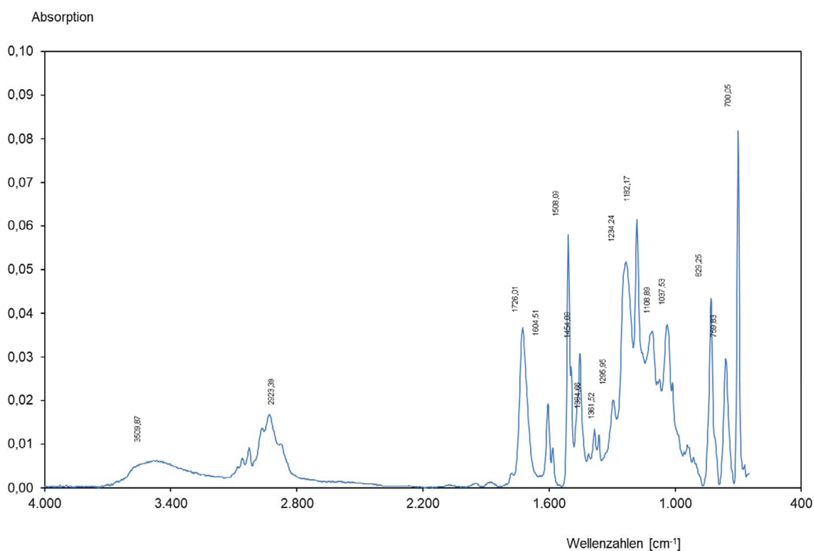
Bild 2: IR-Analyse der Beschichtung
