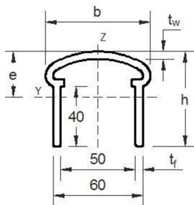
Handlauf 64 x 70
