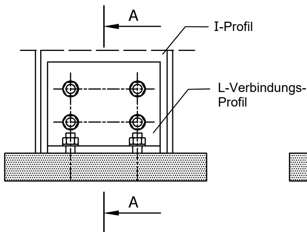
L-Verbindungs-Profil mit Darstellung der einzuhaltenden Lochabstände
