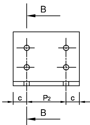
L-Verbindungs-Profil mit Darstellung der einzuhaltenden Lochabstände
