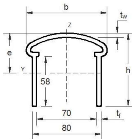
Handlauf 85 x 94
