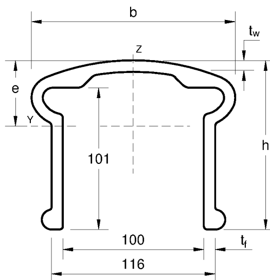
Handlauf 120 x 145
