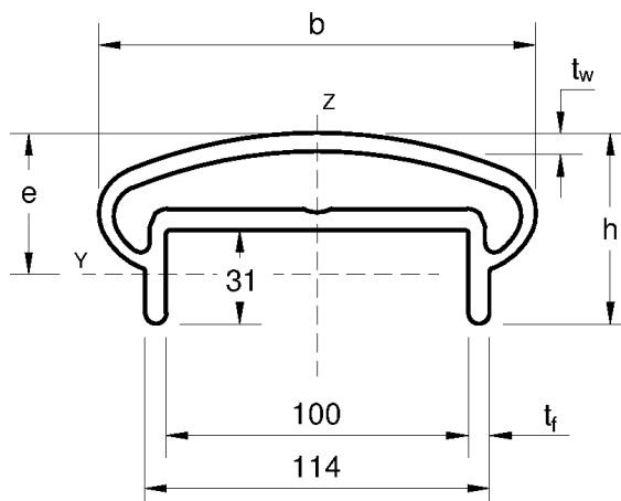
Handlauf 63 x 145
