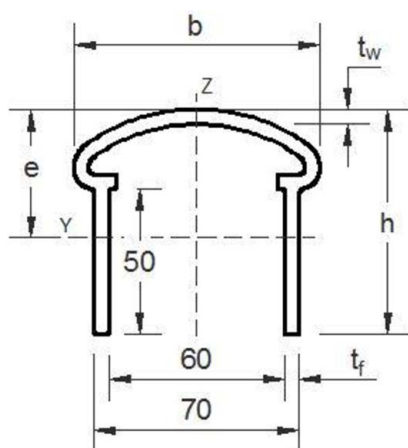
Handlauf 77 x 84
